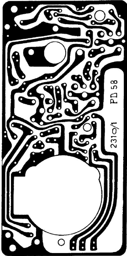
PRANDONI - Mod. NRC22. Apparecchio portatile a transistor, con pannello a circuiti stampati. Antenna magnetica incorporata. Gamma onde medie. Media frequenza a 468 kc/s. Resa d'uscita 200 milliwatt.
