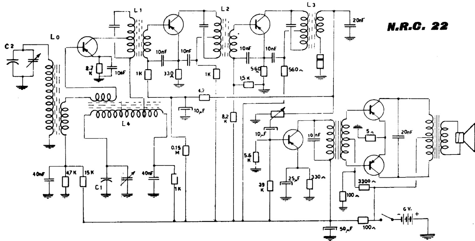
PRANDONI - Mod. NRC22. Apparecchio portatile a transistor, con pannello a circuiti stampati. Antenna magnetica incorporata. Gamma onde medie. Media frequenza a 468 kc/s. Resa d'uscita 200 milliwatt.
